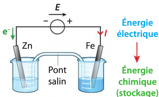
Fonctionnement en électrolyseur
