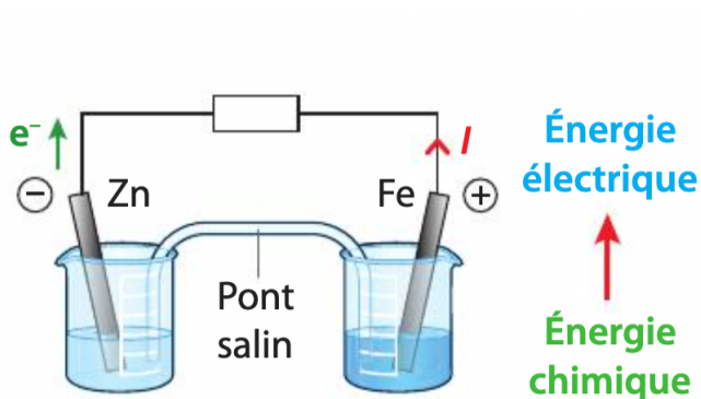
Fonctionnement en pile
